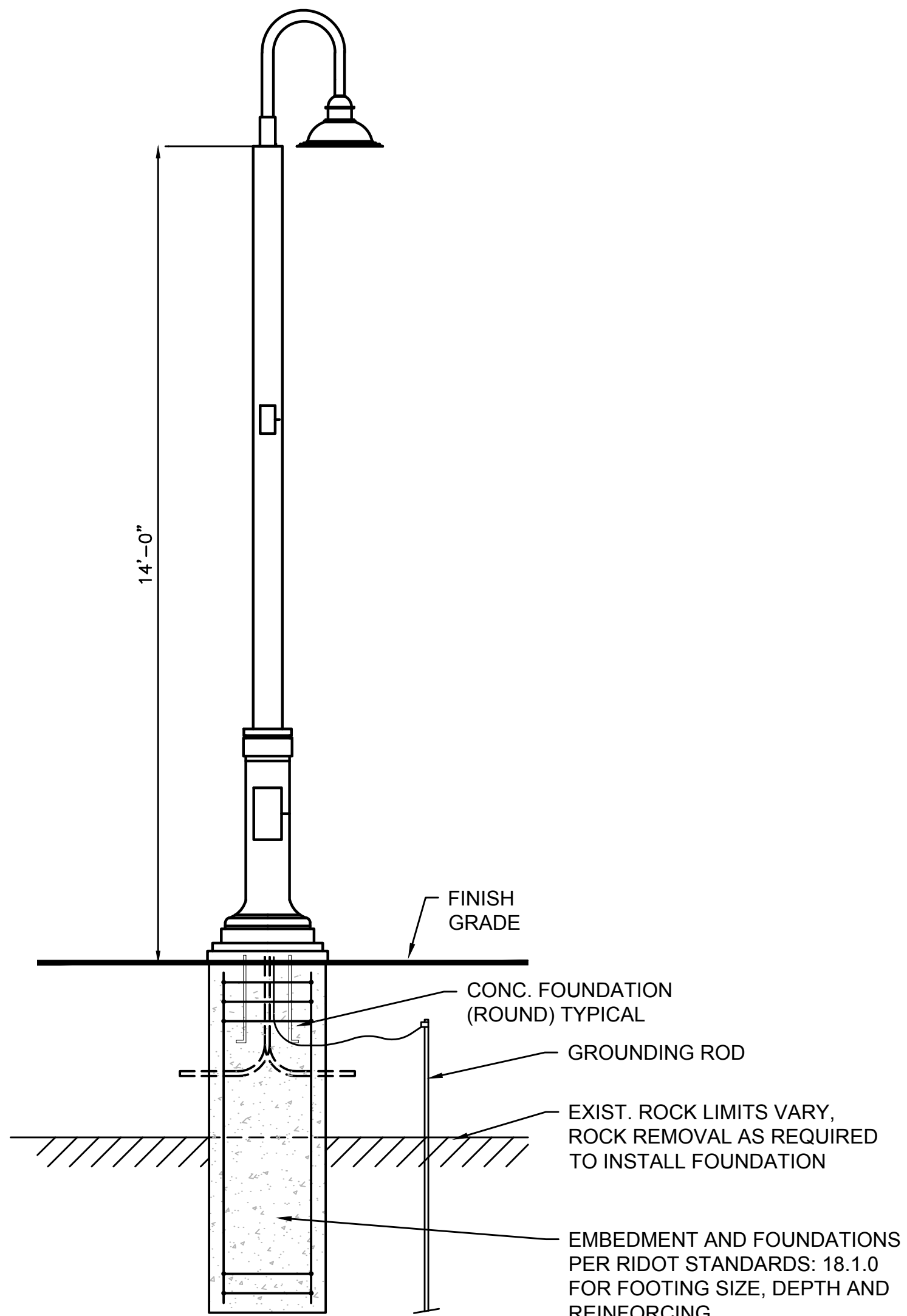
LIGHT TYPE 3 / EC SCALE: 1/2"=1'-0"
